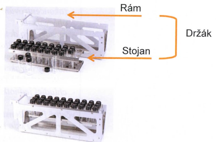
Obrázek č. 2: Držák na sklo se zavěšuje na přední část přístroje
